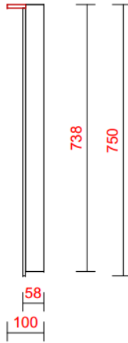
ZIJ-AANZICHT SPIEGEL
