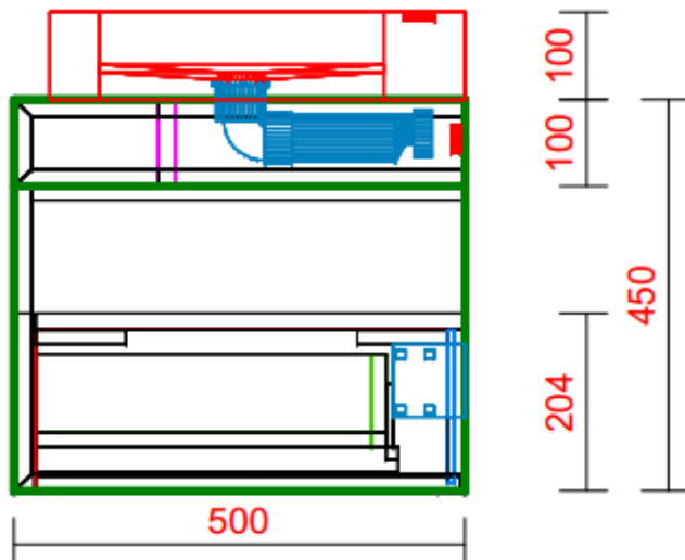
ZIJ-AANZICHT WASTAFEL
