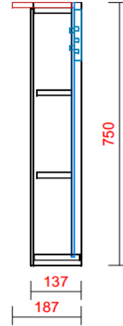
ZIJ-AANZICHT SPIEGELKAST
