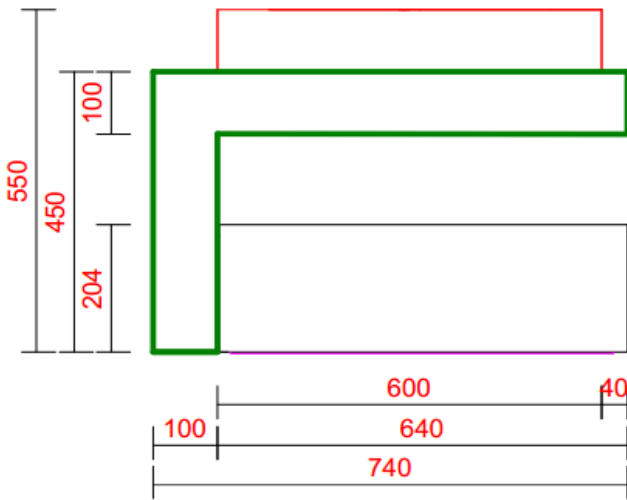
WASTAFEL VOOR-AANZICHT UITVOERING: RECHTS
