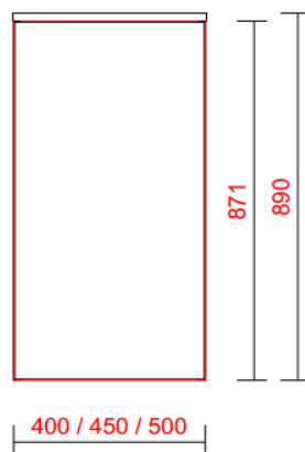
VOOR-AANZICHT
