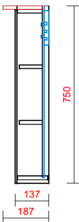
ZIJ-AANZICHT SPIEGELKAST
