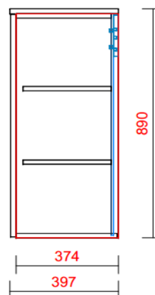
ZIJ-AANZICHT
