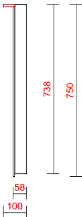
ZIJ-AANZICHT SPIEGEL
