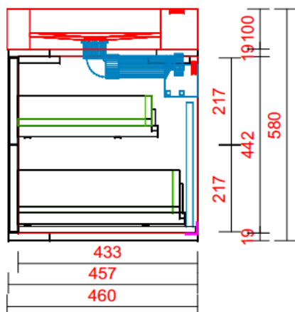
WASTAFEL ZIJ-AANZICHT
