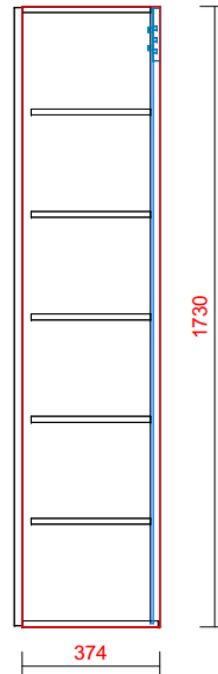
ZIJ-AANZICHT KOLOMKAST
