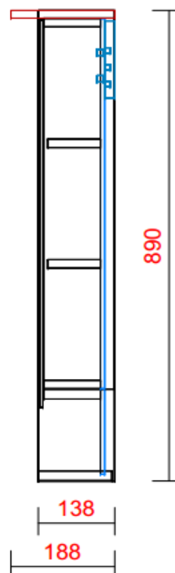
ZIJ-AANZICHT SPIEGELKAST MET REGAAL
