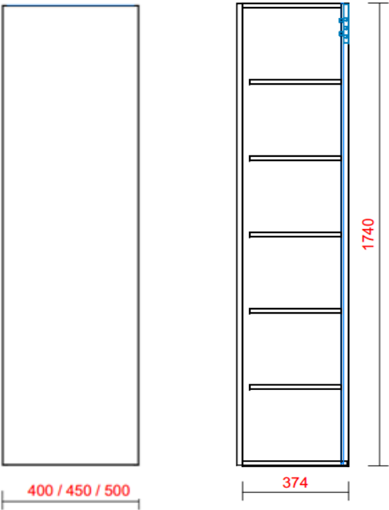
VOOR-AANZICHT KOLOMKAST
