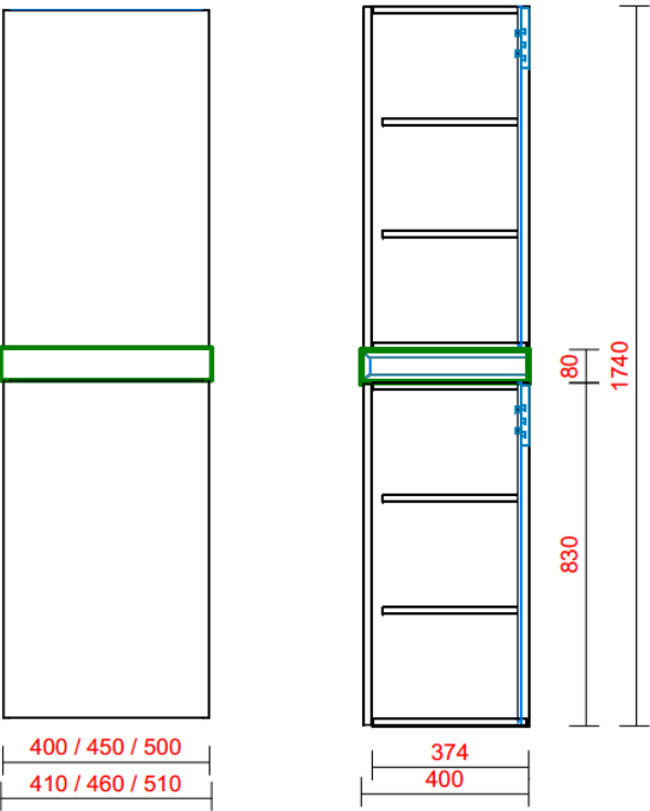
VOOR-AANZICHT KOLOMKAST
