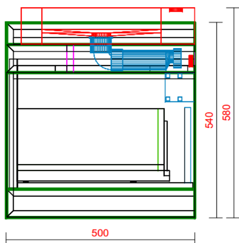
ZIJ-AANZICHT WASTAFEL
