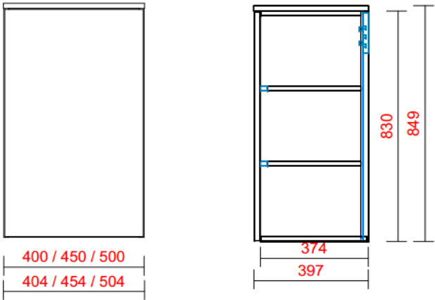
VOOR-AANZICHT KOLOMKAST MET ELEMENT
