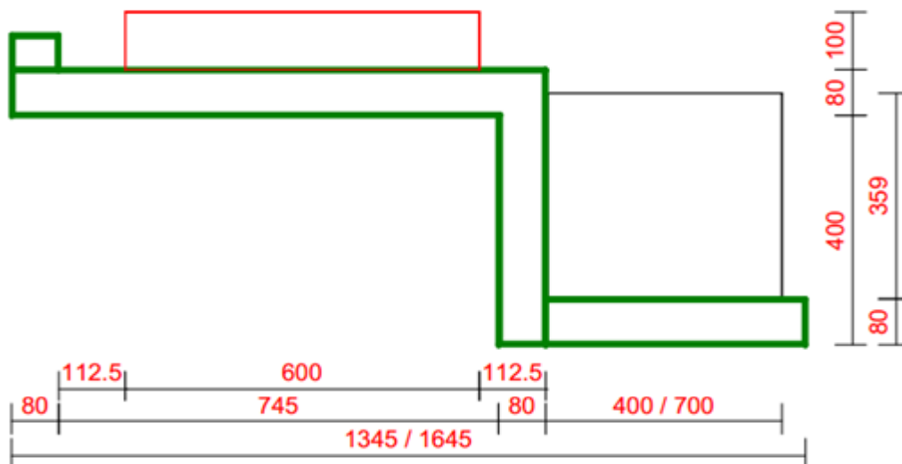
WASTAFEL VOOR-AANZICHT (RECHTS)
