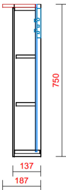
ZIJ-AANZICHT SPIEGELKAST
