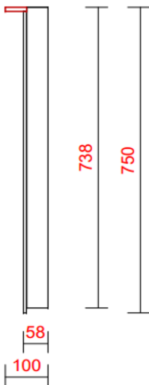
ZIJ-AANZICHT SPIEGEL
